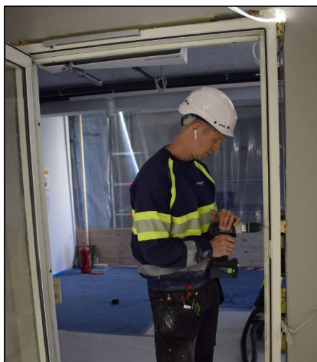
1-2: Dørfelt fra DEG8, overliggende glassfelt fjernet og dør montert i KA13 med ny låssylinder. Foto: Anne S Nordby 3: Brukt brannndør, ferdig montert og lakkert. Foto: Rune Andersen
