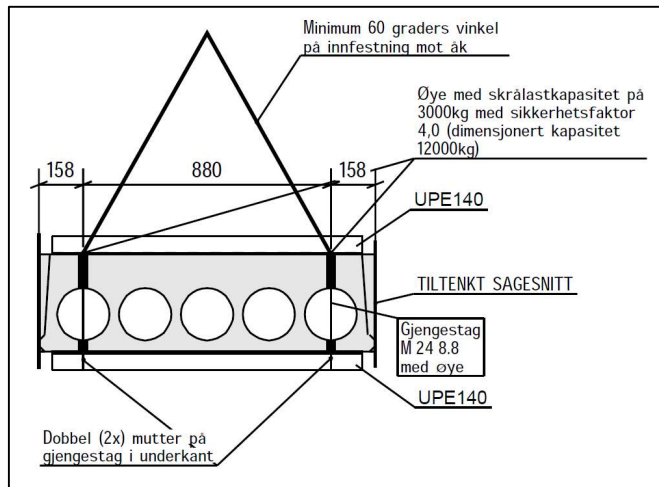
Løfteåk for hulldekkeelementer. Arbeidsteigning, Rambøll.
