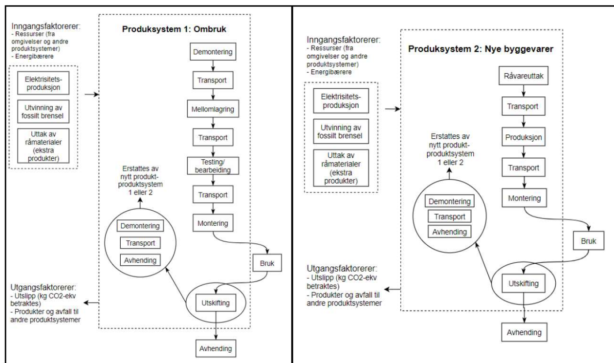
Flytskjema for analyserte produktsystemer. Systemgrensen er markert med stiplet linje (Høydahl og Walter 2020).
