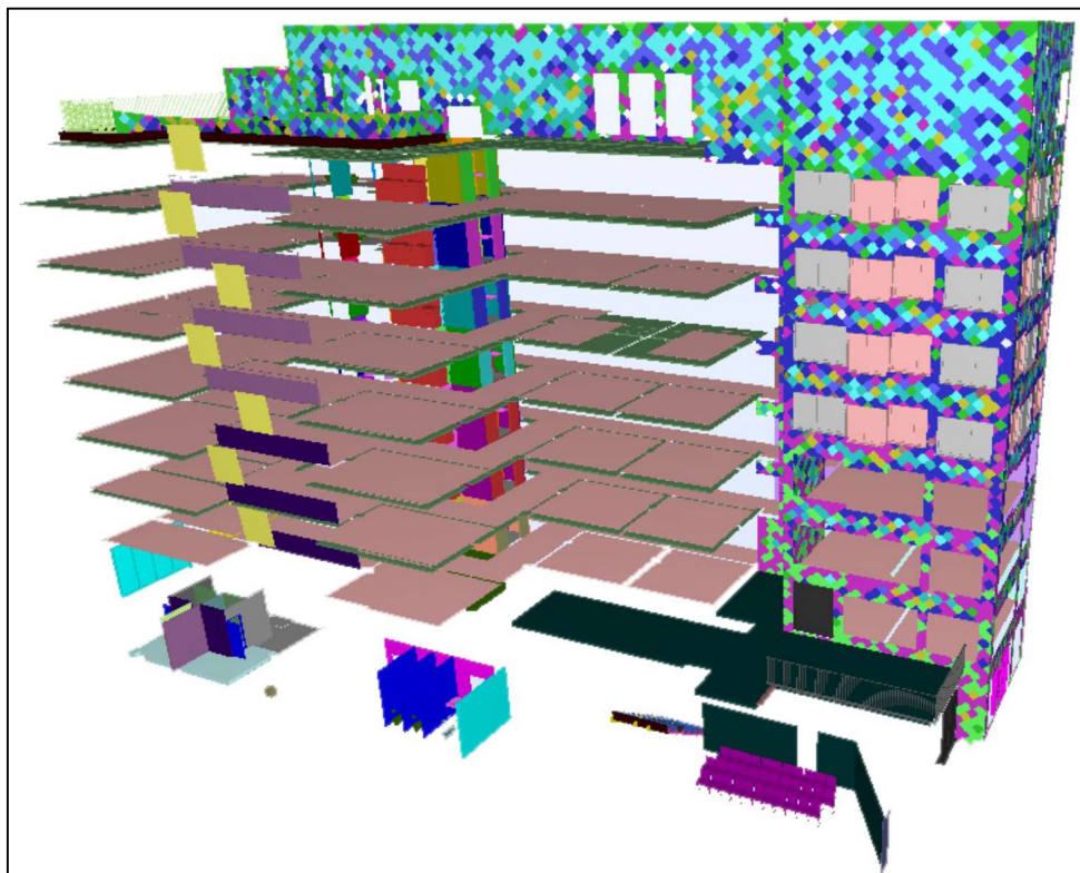
Ombrukte elementer i KA13: Arkitektfaglig og interiør. Bilde fra IFC filen. Illustrasjon: Mad arkitekter
