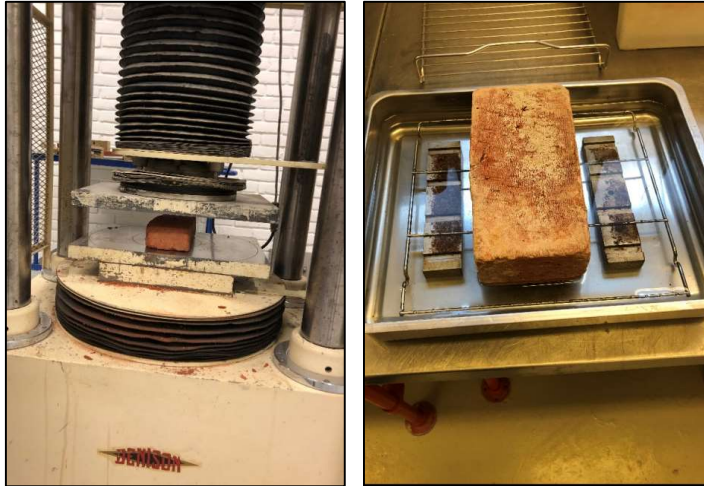
Testing hos Sintef i Oslo; hhv. trykkprøving og minuttsg. Foto: Sintef
