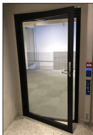
1-2: Dørfelt fra DEG8, overliggende glassfelt fjernet og dør montert i KA13 med ny låssylinder. Foto: Anne S Nordby 3: Brukt brannndør, ferdig montert og lakkert. Foto: Rune Andersen
