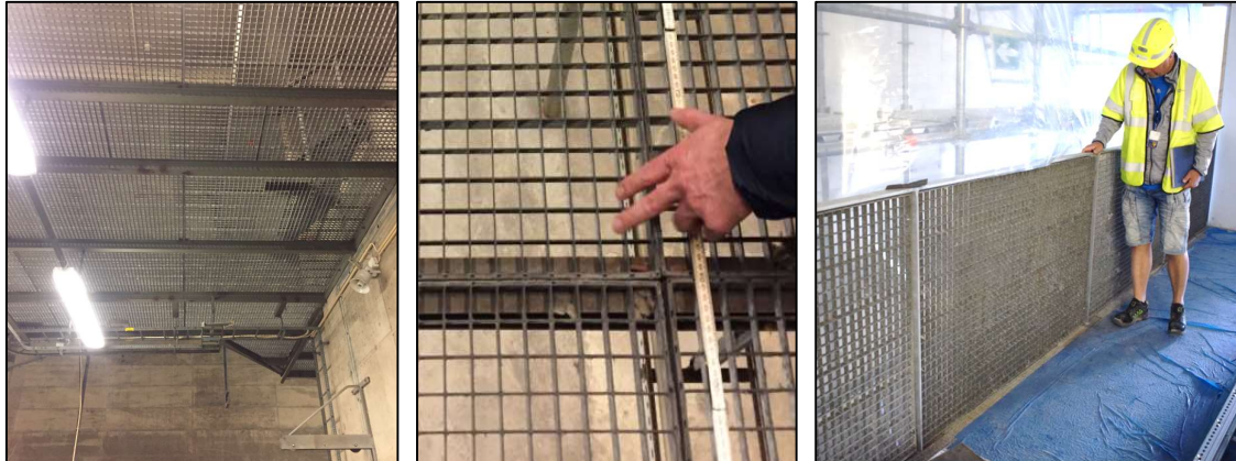
1-2: Gitterrister som gulv i teknisk rom på Tøyenbadet, og oppmåling av disse under befaring. Foto: Catriona Shine.
